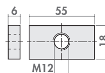
Piastrina zincata a 1 foro
