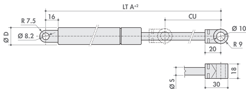
Molla a gas - attacco grosso
