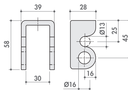
Supporto forato
