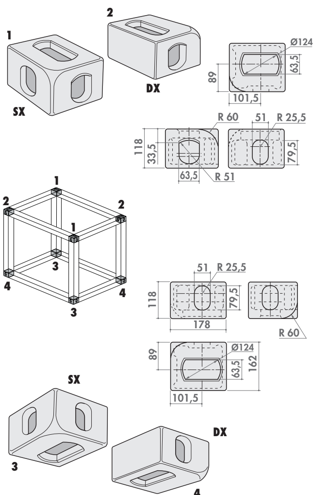
Blocchi angolari per containers
