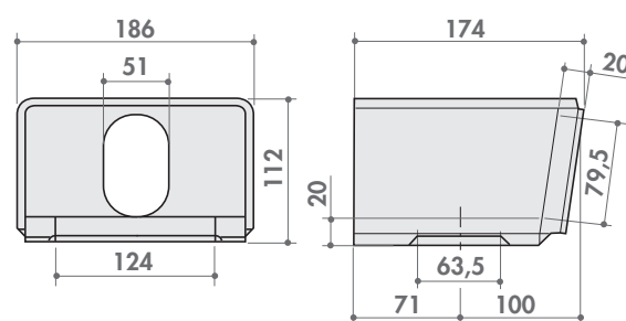
Blocco d'angolo inclinato per scarrabili
