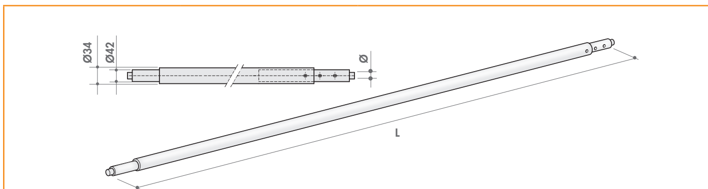
Barra fermacarico telescopica in acciaio zincato
