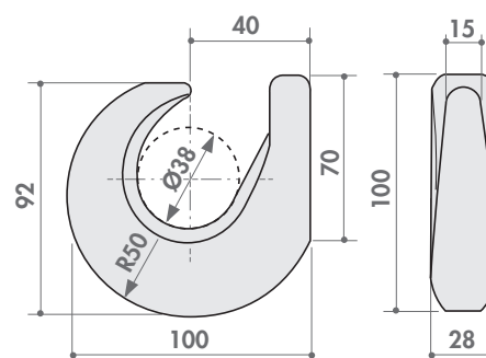
Gancio traino medio
