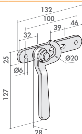
Tendicatena esterno
