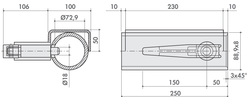
Supporto rigido da 80 mm
