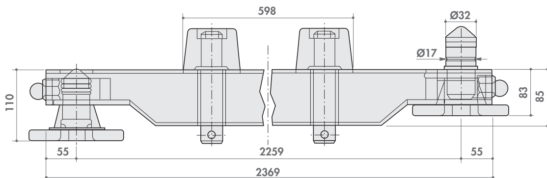
Traversa con twist e rulli 85x160 mm
