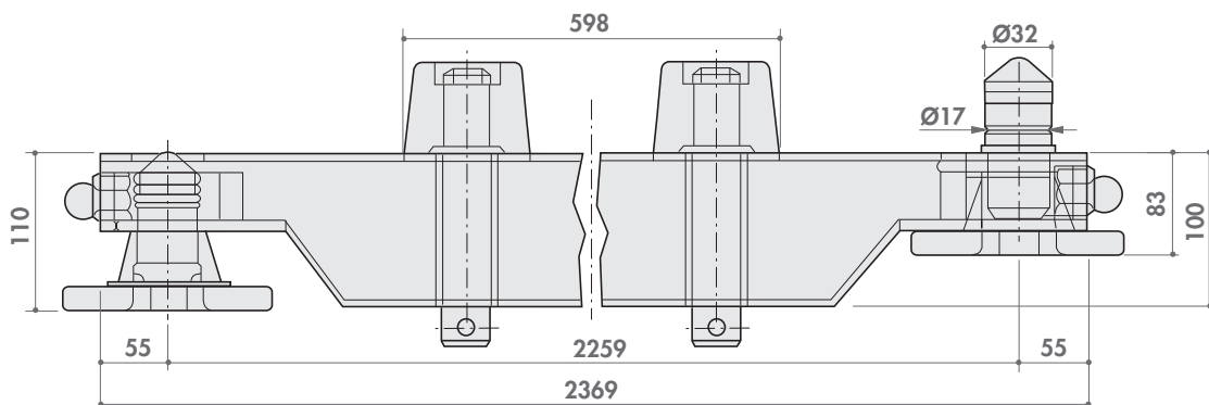
Traversa con twist e rulli 100x200 mm
