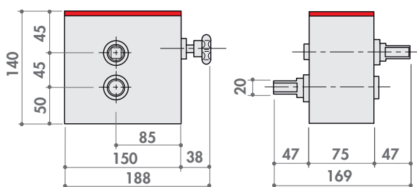
Riduttore per centina CESCHI 1 a 4
