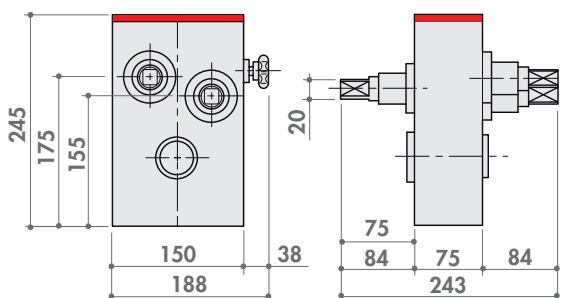
Riduttore per centina CESCHI 1 a 8 - 1 a 16
