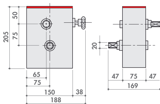
Riduttore per centina CESCHI 1 a 8
