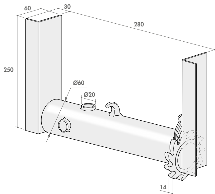
Verricello Ø60 mm rinforzato destro e sinistro
