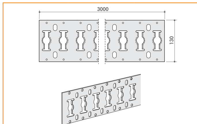
Profilo piatto fermacarico mt. 2.964
