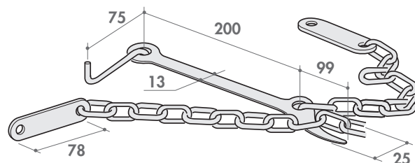
Serie catena zincata completa
