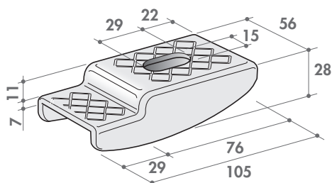
Staffa anti sdrucchiolo zincata piccola
