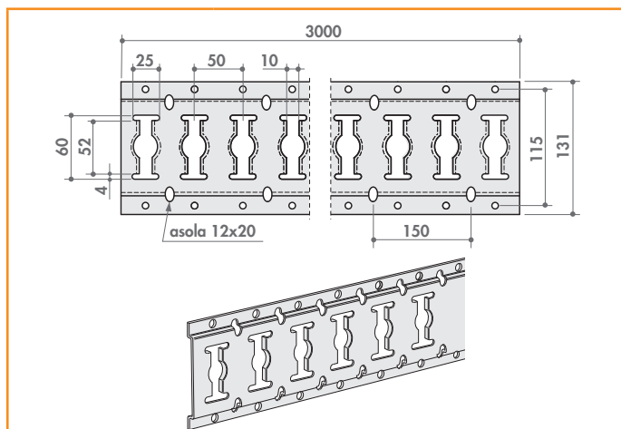
Profilo fermacarico mt. 3
