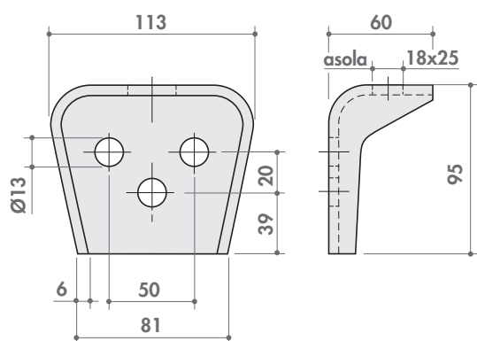
Supporto telaio 190 corto
