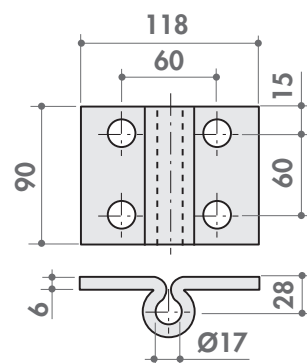
Supporto tipo 330 grezzo
