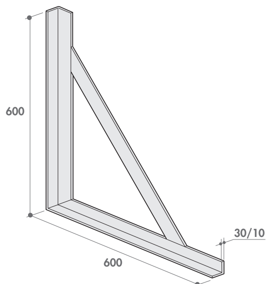
Staffa pesante zincata
