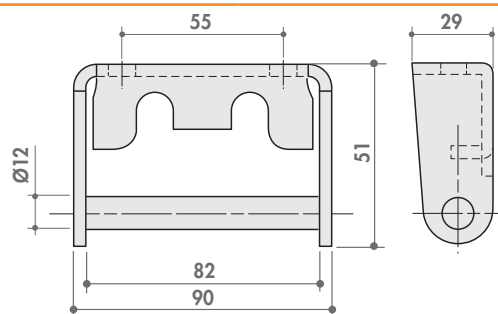
Cerniera "Viberti" maschio
