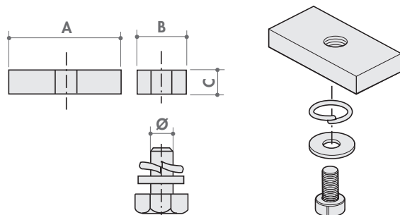
Kit fissaggio paraciclisti
