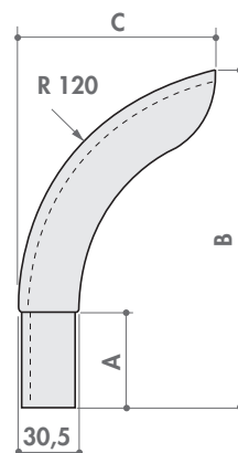
Tappo in PVC per profilo anteriore
