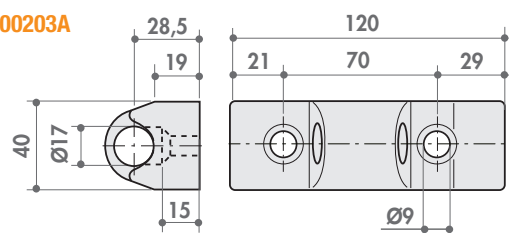
Cerniera tir pesante
