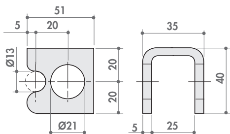
Supporto forato leggero Ø21 mm
