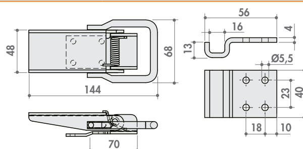
Anello piccolo con nottolino
