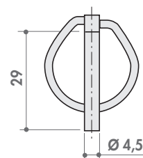
Coppiglia mm 4,4
