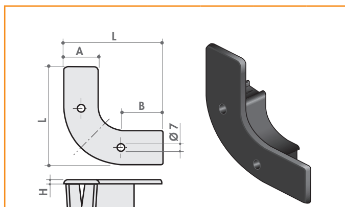
Tappo posteriore mod. PR in PVC nero
