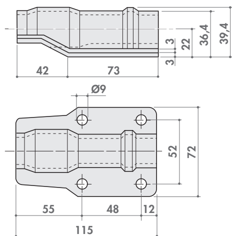
Supporto guida mm 39 zincato
