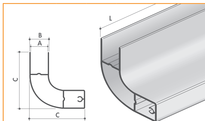
Profilo angolare in alluminio
