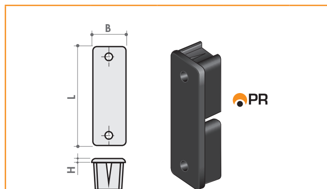
Tappo posteriore mod. PR in PVC nero
