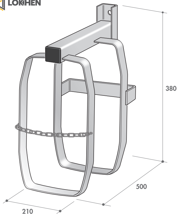
Supporto per tanica
