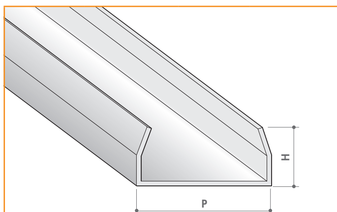
Lama per tampone - L 2600 mm
