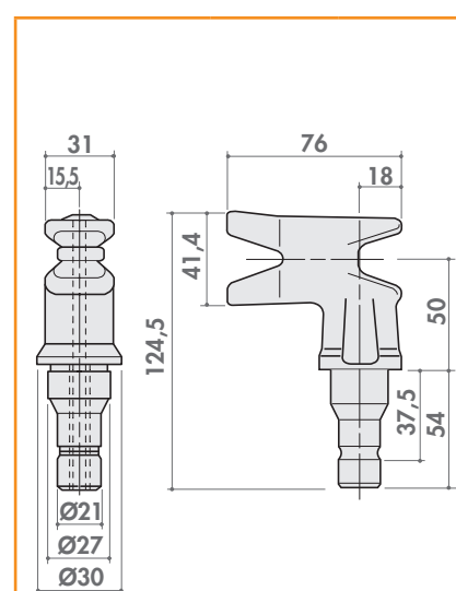
Arpione chiusura Ø27 mm
