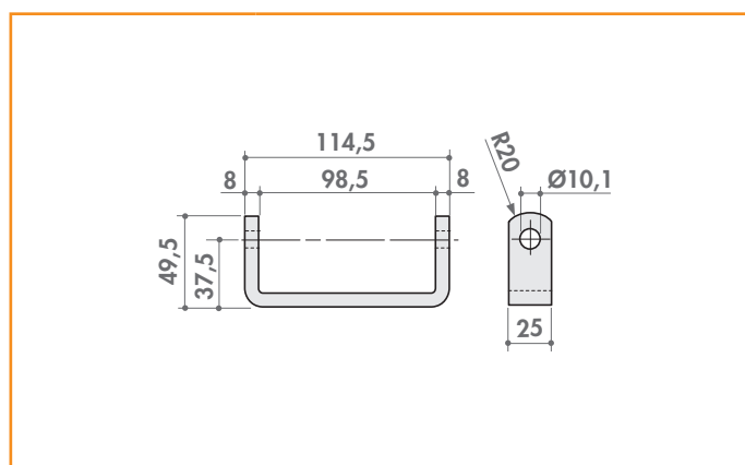
Cavallotto H 37,5 mm - L 114,5 mm
