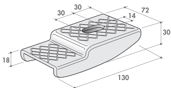
Staffa anti sdrucchio zincata grande
