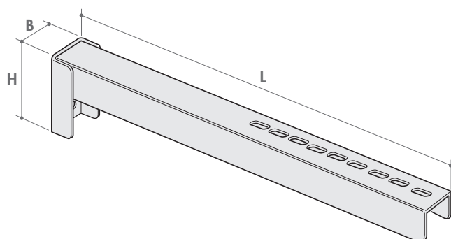
Staffa asolata grezza per supporto ancoraggio paraciclisti
