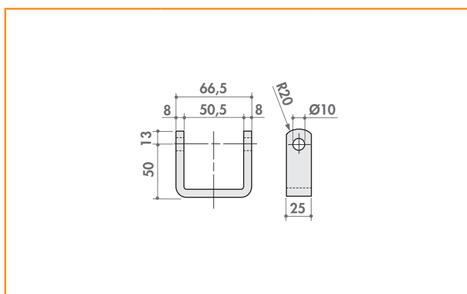
Cavallotto H 50 mm
