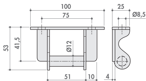
Cerniera sponda ribaltabile leggera
