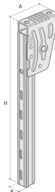
Ancoraggio paraciclisti
