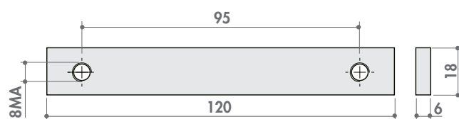
Piastrina zincata interasse 95 mm - 120x18x6 mm
