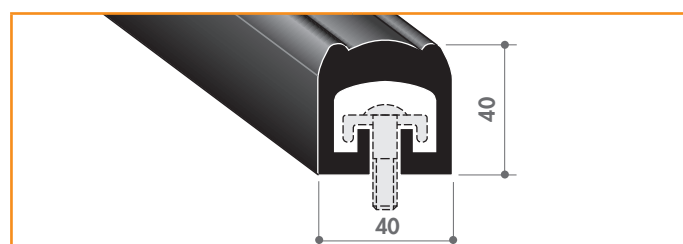
Tampone in PVC - L 2600 mm (lama zincata esclusa)
