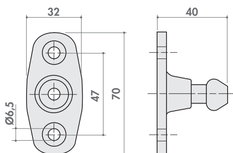
Perno fermaporta mm 40
