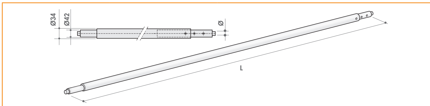
Barra fermacarico telescopica in acciaio zincato
